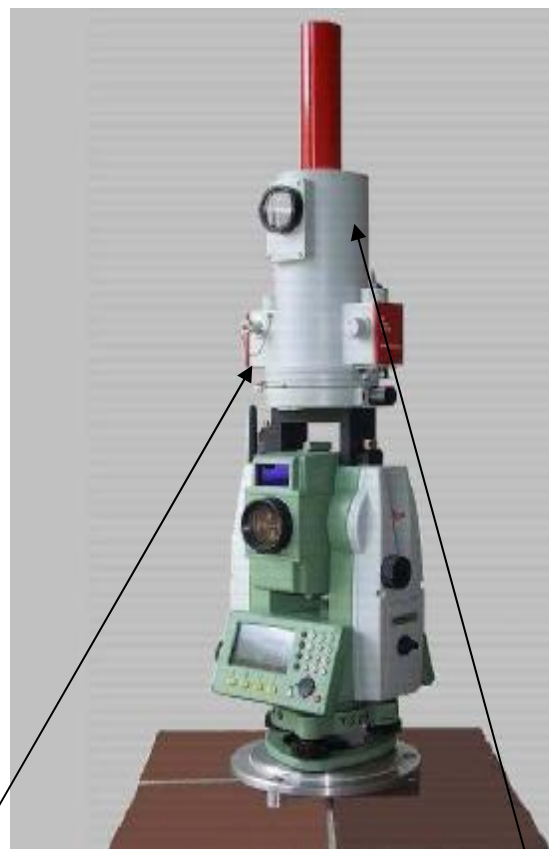
Рисунок 2 – Вид гиронасадки со стороны объектива а – место пломбировки б – место нанесения наклейки со знаком утверждения типа
